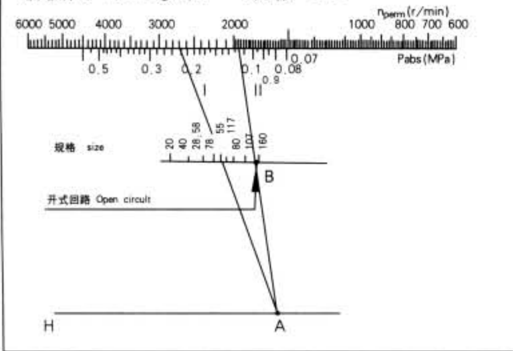
诺模图 Nomograph 规格 Size 170
