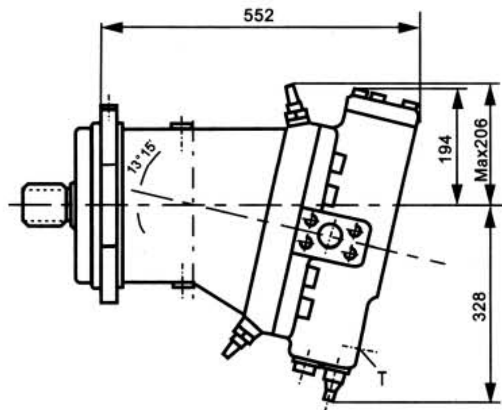
EP电控变量 Electric Control
