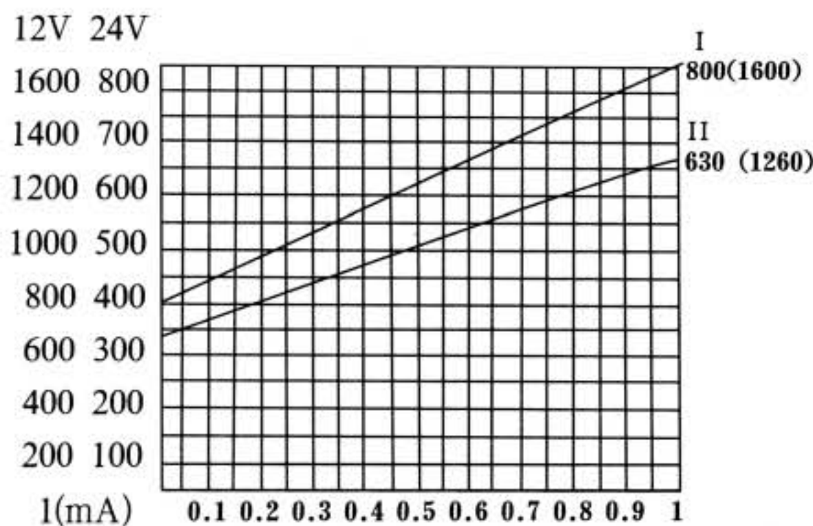
EP 电控比例变量 Electric pro.Control
