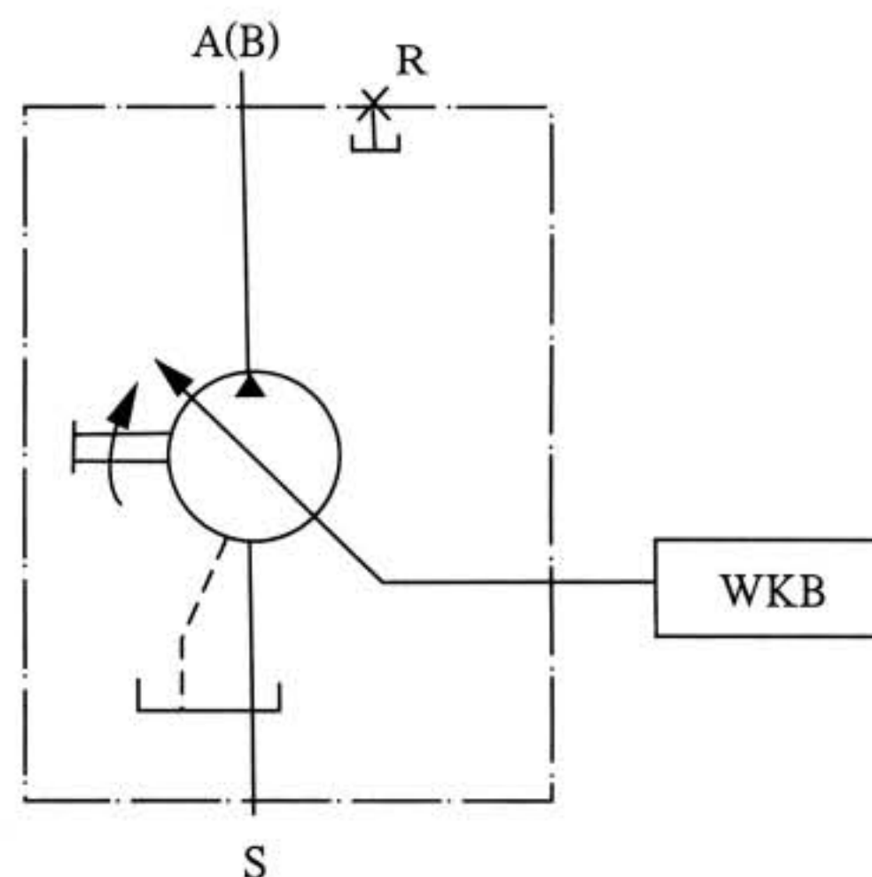
NC数字变量 Numerical control.NC
