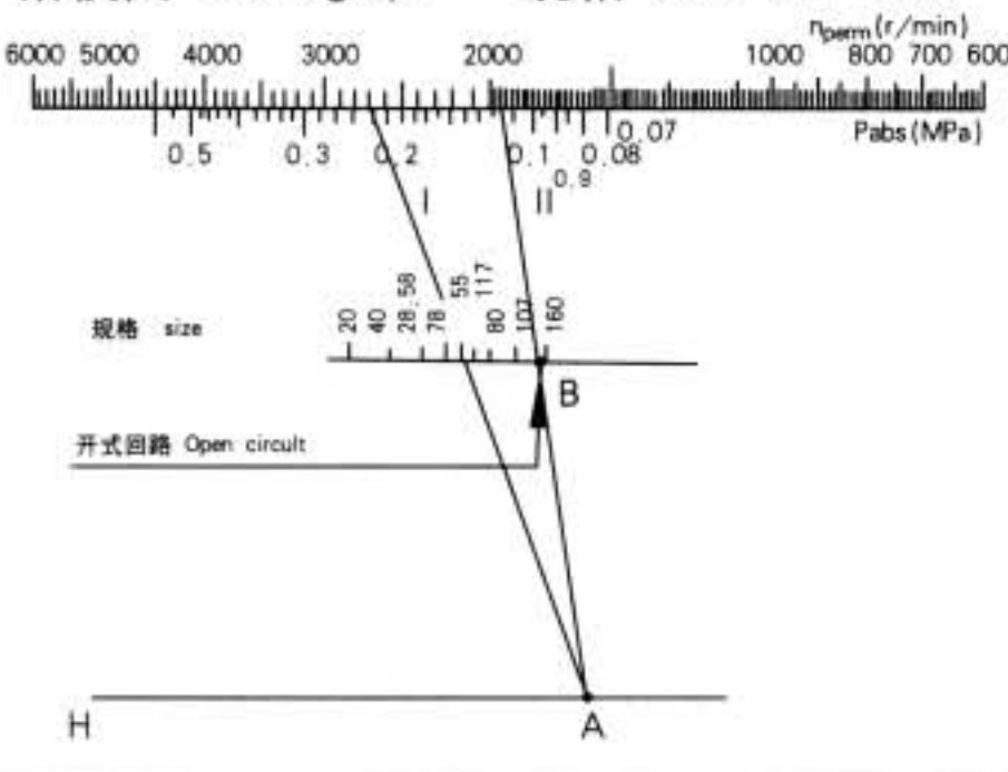
诺模图 Nomograph 规格 Size 20–160
