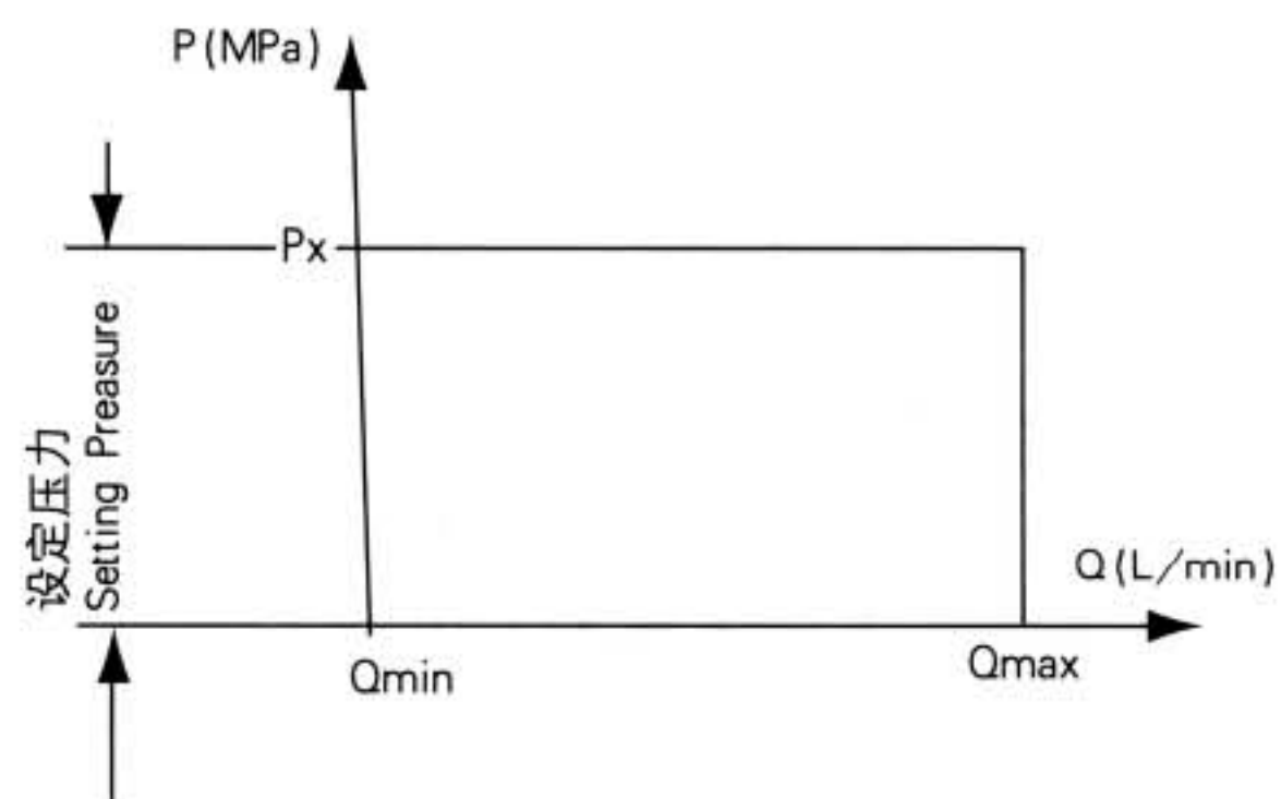
SC的P-Q特性曲线 Characteristics
