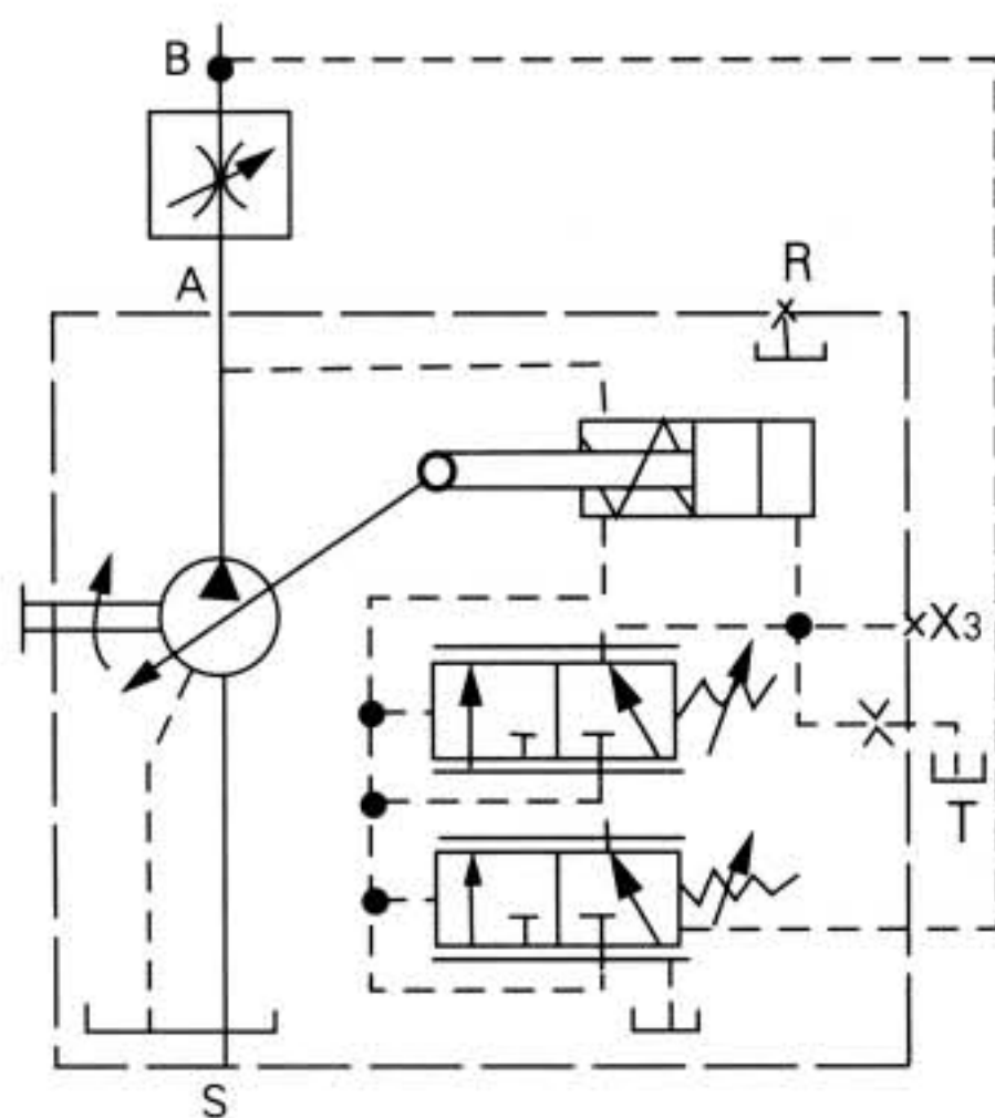
DRS 恒压带负荷传感变量
