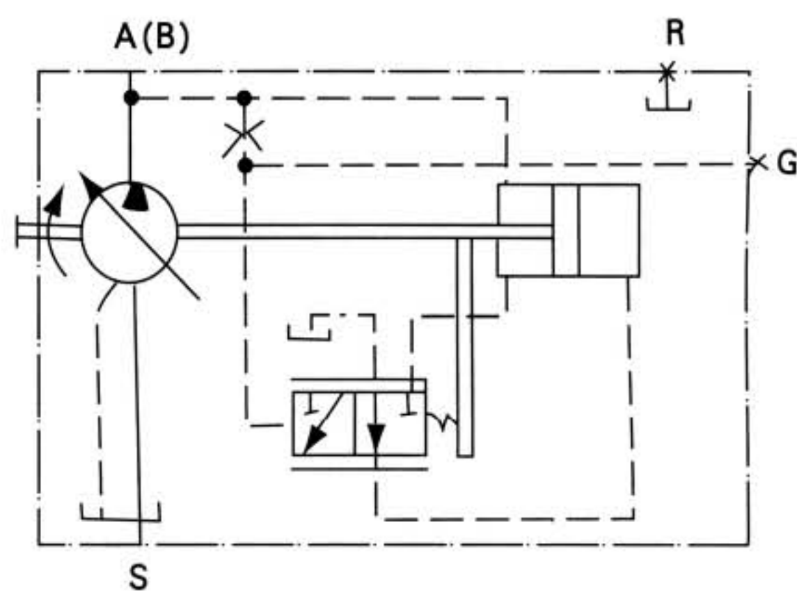
SC刹车变量 Brake control.SC
