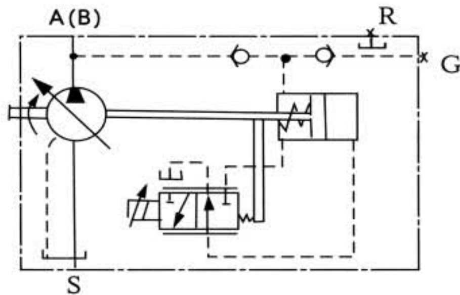
EP 电控比例变量 Electric pro.Control
