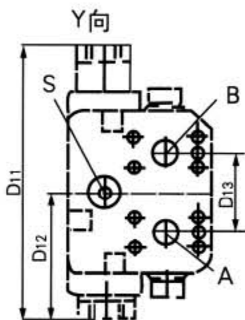
油口接板 17,181 (单级溢流阀)
