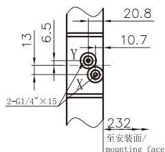
A 的安装尺寸/Dimensions
