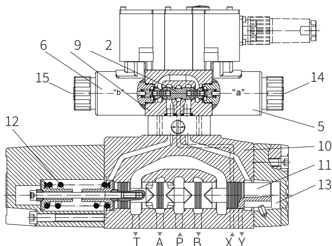
Model 4WRZE16...-7XT/..
